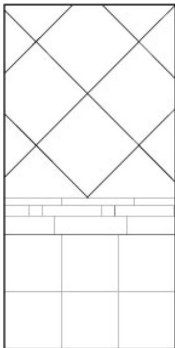
CODICE 223 cm 100,5x201x1,8 FONDO 42,5X42,5 MURETTO 21X42,5 FONDO 33,3X33,3
