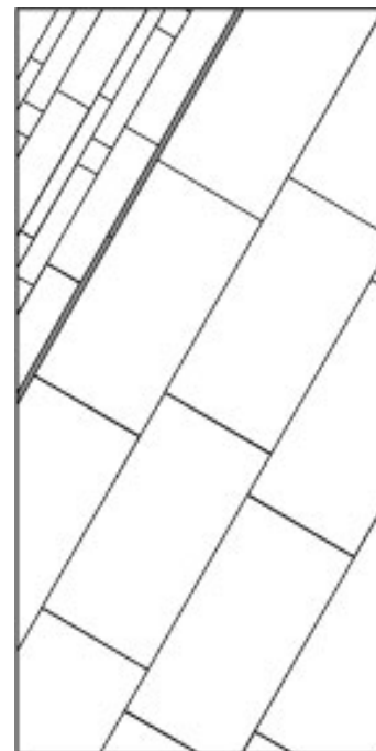
CODICE 237 cm 100,5x201x1,8 MURETTO 21X42,5 LIST.ALLUMINIO 1,5X100 FONDO 33,3X66,6
