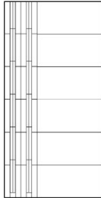
CODICE 201 cm 100,5x201x1,8 FONDO 33,3X66,6 MURETTO 33,3X33,3
