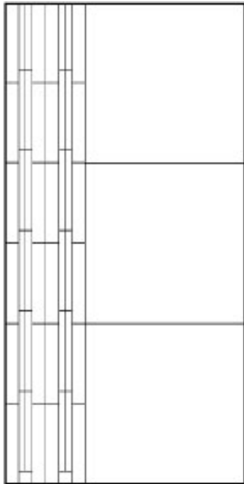
CODICE 200 cm 100,5x201x1,8 FONDO 66,6X66,6 MURETTO 33,3X33,3
