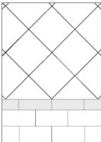
CODICE 051 cm 100,5x140,5x1,4 FONDO 33,3X33,3 FONDO 16,5X33,3 FASCIA **X33,3
