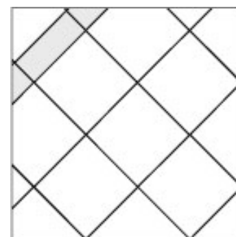
CODICE 384 cm 100,5x100,5x1,2 FONDO 33,3X33,3 FASCIA **X33,3
