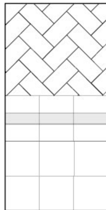
CODICE 284 cm 100,5x201x1,8 FONDO 33,3X33,3 FONDO 16,5X33,3 FASCIA **X33,3
